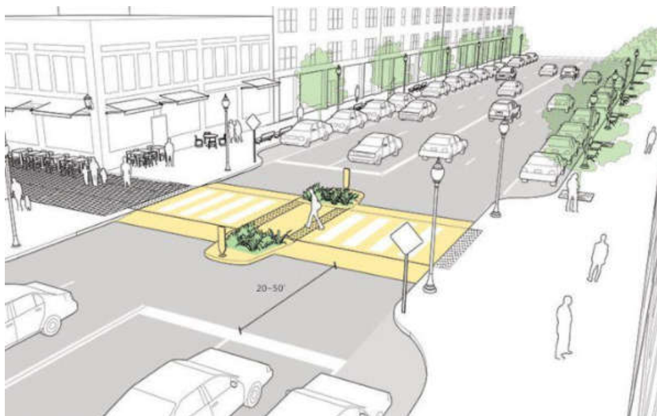
Figura 2.5.67. Traversări mediane – Propunere de ridicare a cotei carosabilului la cea a trotuarului
