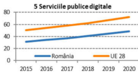
Figura 2.9.22. DESI 2020
