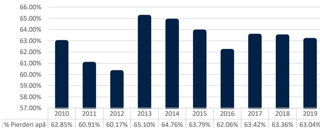
Figura 14. Evoluția pierderilor de apă (%) în Suceava (2010-2019)
