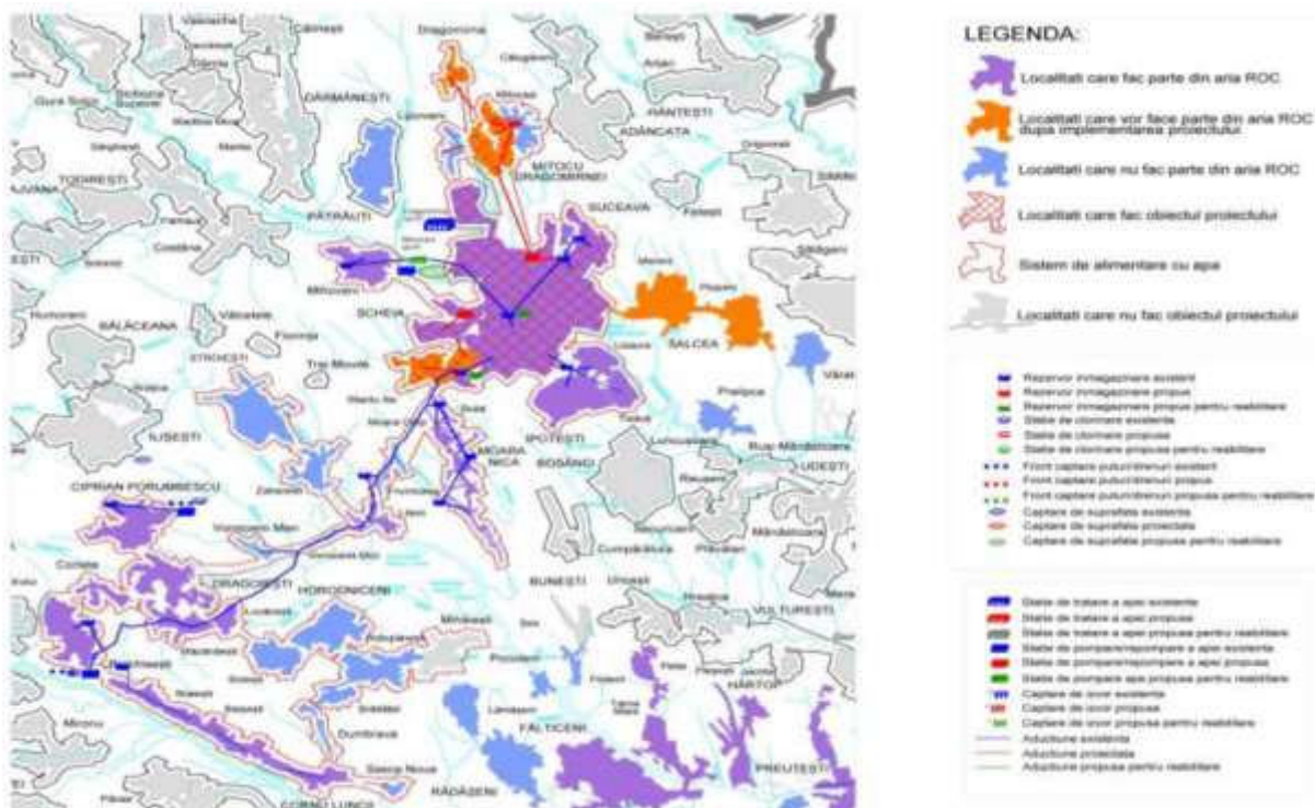
Figura 1. Sistemul de alimentare cu apă Suceava
