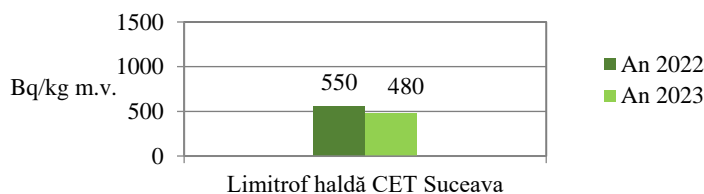
Fig. 2.6.2.1. Vegetație spontană – activități beta globale, în anul 2023, comparativ cu anul 2022 – măsurători la 5 zile de la prelevare
