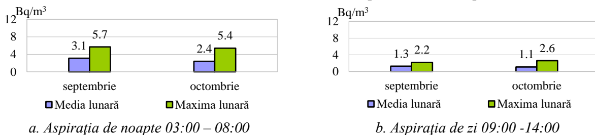
Fig. 2.2.1.1. Aerosoli atmosferici, activități specifice beta globale imediate – valori medii și maxime în luna octombrie 2023, comparativ cu luna septembrie 2023
