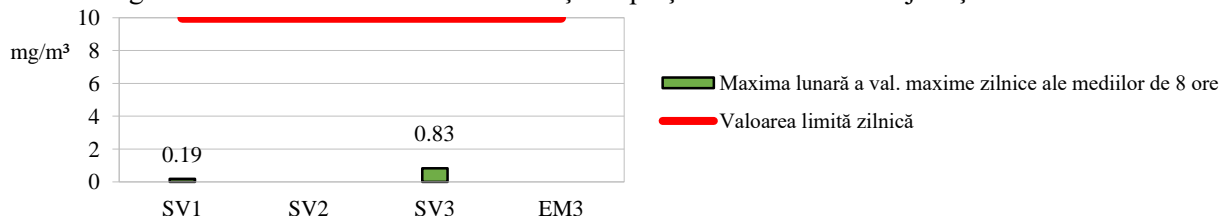
Fig. 1.3.2. Concentrații maxime lunare ale mediilor de 8 ore de CO înregistrate în luna octombrie 2023 la stațiile aparținând RNMCA din județul Suceava
