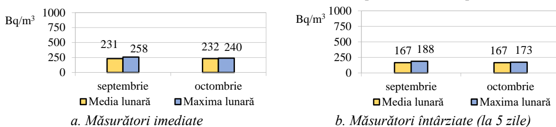
Fig. 2.4.1.1. Apă brută (râu Suceava - Burdujeni), activități specifice beta globale imediate și întârziate - medii lunare și maxime zilnice în luna octombrie 2023, comparativ cu luna septembrie 2023
