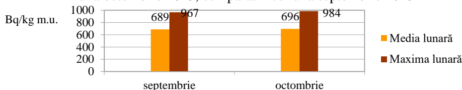
Fig. 2.5.1.1. Sol necultivat mun. Suceava - activități specifice beta globale întârziate în luna octombrie 2023, comparativ cu luna septembrie 2023
