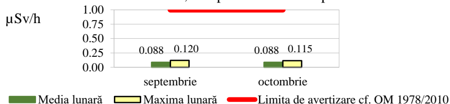
Fig. 2.1.1. Debitul dozei gamma în aer ( \mu\text{Sv/h} ) - medii și maxime în luna octombrie 2023, comparativ cu luna septembrie 2023
