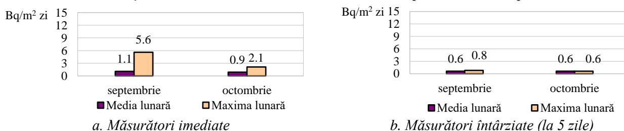
Fig. 2.3.1. Depuneri atmosferice, activități specifice beta globale imediate și întârziate (la 5 zile) - medii lunare și maxime zilnice în luna octombrie 2023, comparativ cu luna septembrie 2023
