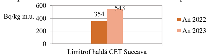
Fig. 2.5.2.1. Sol necultivat – activități beta globale, în anul 2023, comparativ cu anul 2022 – măsurători la 5 zile de la prelevare
