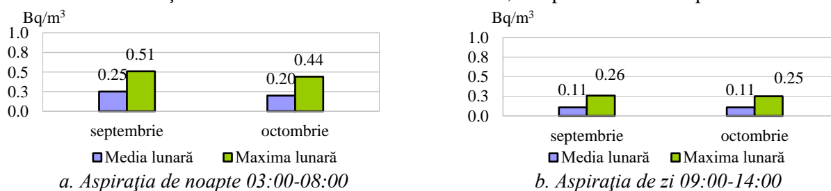
Fig. 2.2.2.2. Activități specifice ale Toronului ( Rn-220 ) în atmosfera liberă - medii lunare și maxime zilnice în luna octombrie 2023, comparativ cu luna septembrie 2023
