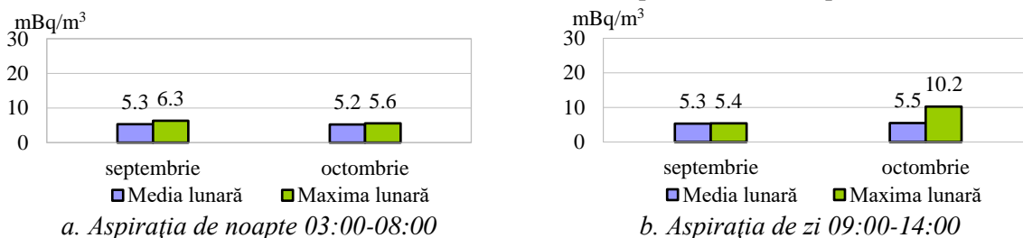
Fig. 2.2.3.1. Aerosoli atmosferici, activități specifice beta globale întârziate (la 5 zile) - valori medii și maxime în luna octombrie 2023, comparativ cu luna septembrie 2023
