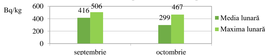
Fig. 2.6.1.1. Vegetație spontană mun. Suceava - activități specifice beta globale întârziate în luna octombrie 2023, comparativ cu luna septembrie 2023
