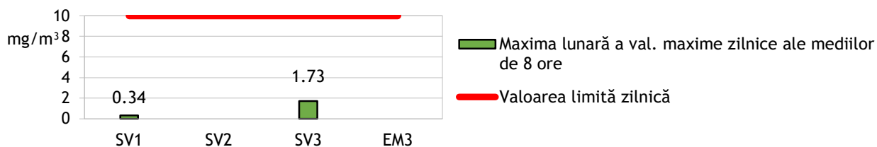
Fig. 1.3.2. Concentrații maxime lunare ale mediilor de 8 ore de CO înregistrate în luna martie 2024 la stațiile aparținând RNMCA din județul Suceava
