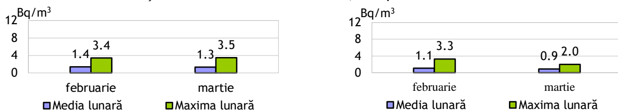
Fig. 2.2.1.1. Aerosoli atmosferici, activități specifice beta globale imediate - valori medii și maxime în luna martie 2024, comparativ cu februarie 2024
