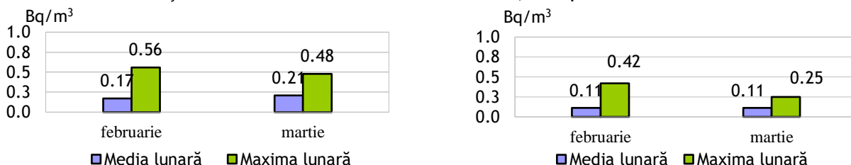
Fig. 2.2.2.2. Activități specifice ale Toronului (Rn-220) în atmosfera liberă - medii lunare și maxime zilnice în luna martie 2024, comparativ cu luna februarie 2024
