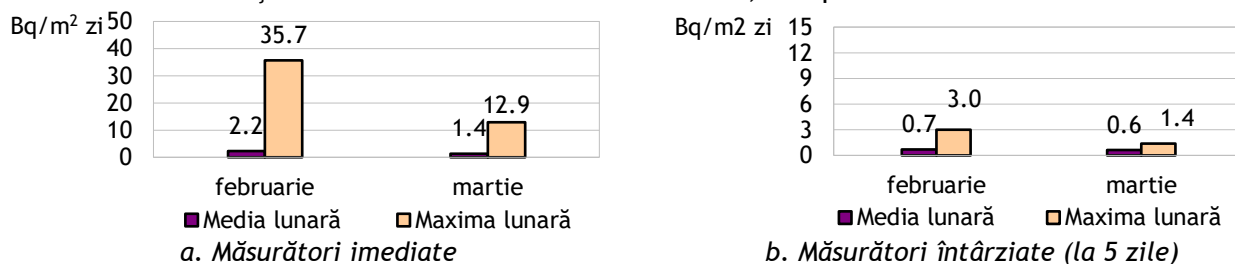
Fig. 2.3.1. Depuneri atmosferice, activități specifice beta globale imediate și întârziate (la 5 zile) - medii lunare și maxime zilnice în luna martie 2024, comparativ cu luna februarie 2024
