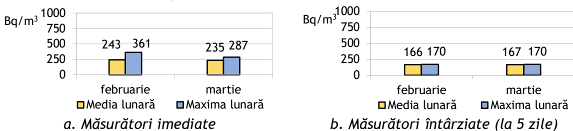
Fig. 2.4.1.1. Apă brută (râu Suceava - Burdujeni), activități specifice beta globale imediate și întârziate - medii lunare și maxime zilnice în martie 2024, comparativ cu februarie 2024
