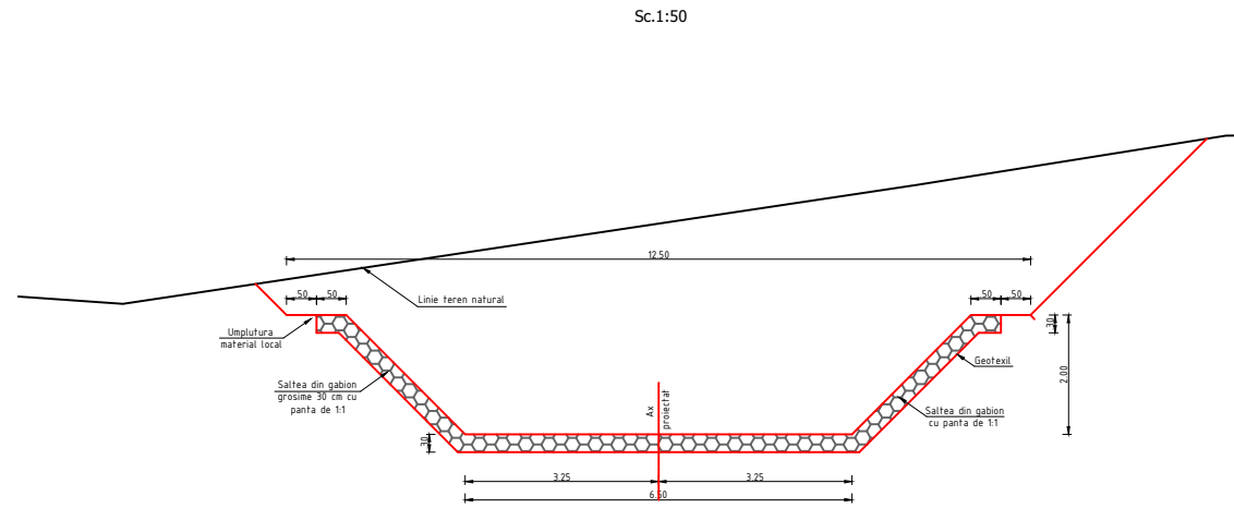
PROTECTIE ALBIE CU SALTEA DE GABIOANE
