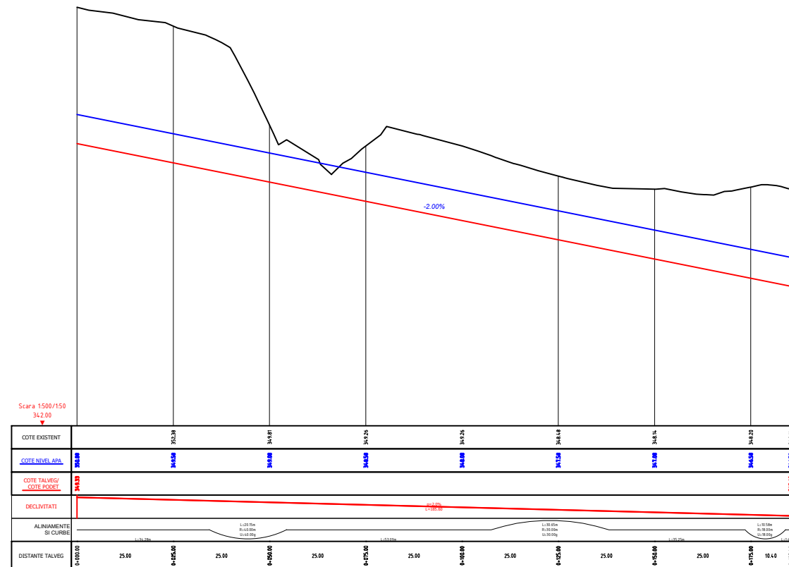
PROFIL LONGITUDINAL
