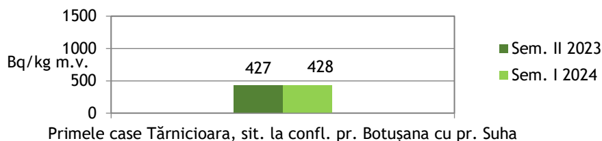
Fig. 2.6.2.1. Vegetație spontană - activitate beta globală, în sem. I 2024, comparativ cu sem. II 2023 - măsurători la 5 zile de la prelevare
