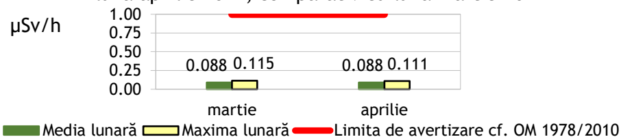
Fig. 2.1.1. Debitul dozei gamma în aer (µSv/h) - medii și maxime în luna aprilie 2024, comparativ cu luna martie 2024
