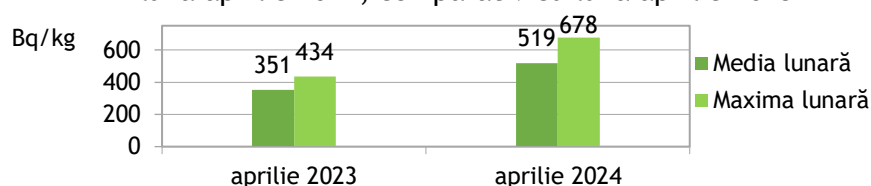
Fig. 2.6.1.1. Vegetație spontană mun. Suceava - activități specifice beta globale întârziate în luna aprilie 2024, comparativ cu luna aprilie 2023
