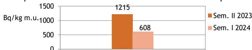
Fig. 2.5.2.1. Sol necultivat - activitate beta globală, în sem. I 2024, comparativ cu sem. II 2023 - măsurători la 5 zile de la prelevare
