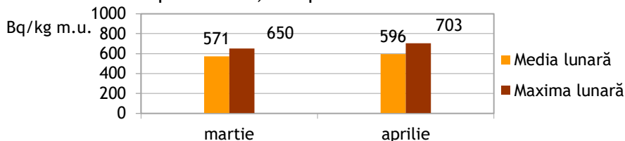
Fig. 2.5.1.1. Sol necultivat mun. Suceava - activități specifice beta globale întârziate în luna aprilie 2024, comparativ cu luna martie 2024
