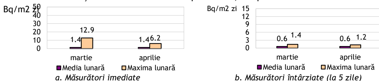
Fig. 2.3.1. Depuneri atmosferice, activități specifice beta globale imediate și întârziate (la 5 zile) - medii lunare și maxime zilnice în luna aprilie 2024, comparativ cu luna martie 2024
