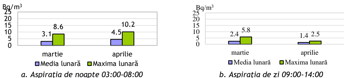
Fig. 2.2.2.1. Activități specifice ale Radonului (Rn-222) în atmosfera liberă - valori medii și maxime în luna aprilie 2024, comparativ cu luna martie 2024
