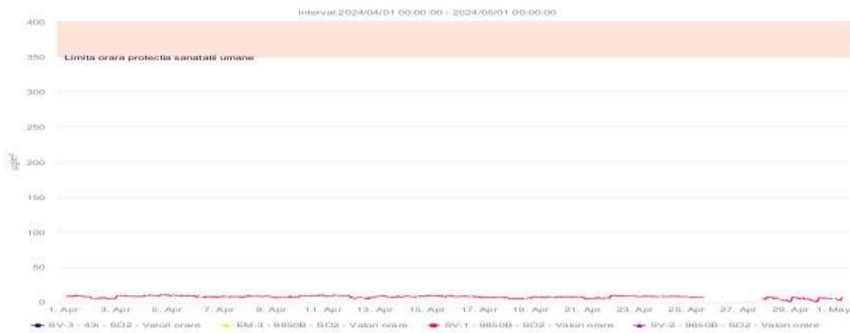
Fig. 1.5.1. Evoluția concentrațiilor medii orare de \text{SO}_2 înregistrate în luna aprilie 2024 la stațiile aparținând RNMCA din județul Suceava
