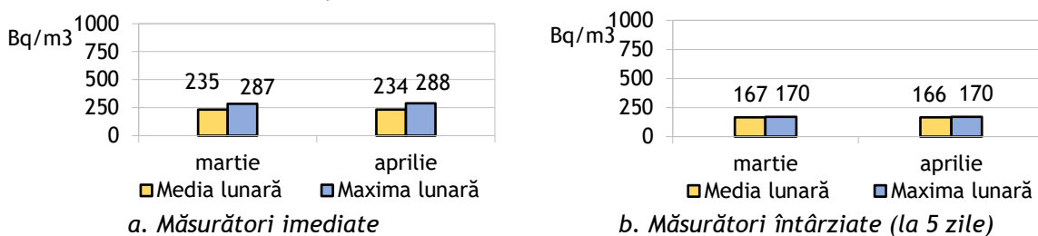
Fig. 2.4.1.1. Apă brută (râu Suceava - Burdujeni), activități specifice beta globale imediate și întârziate - medii lunare și maxime zilnice în aprilie 2024, comparativ cu martie 2024
