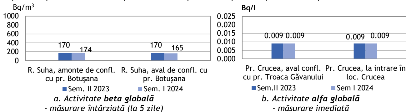
Fig. 2.4.2.1. Apă de suprafață - activități beta și alfa globale
