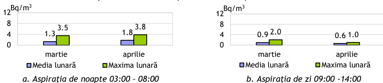
Fig. 2.2.1.1. Aerosoli atmosferici, activități specifice beta globale imediate - valori medii și maxime în luna aprilie 2024, comparativ cu martie 2024
