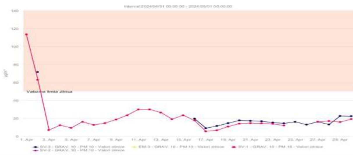
Fig. 1.1.1. Evoluția concentrațiilor medii zilnice la particule în suspensie PM10 determinate gravimetric în luna aprilie 2024, la stațiile aparținând RNMCA din județul Suceava
