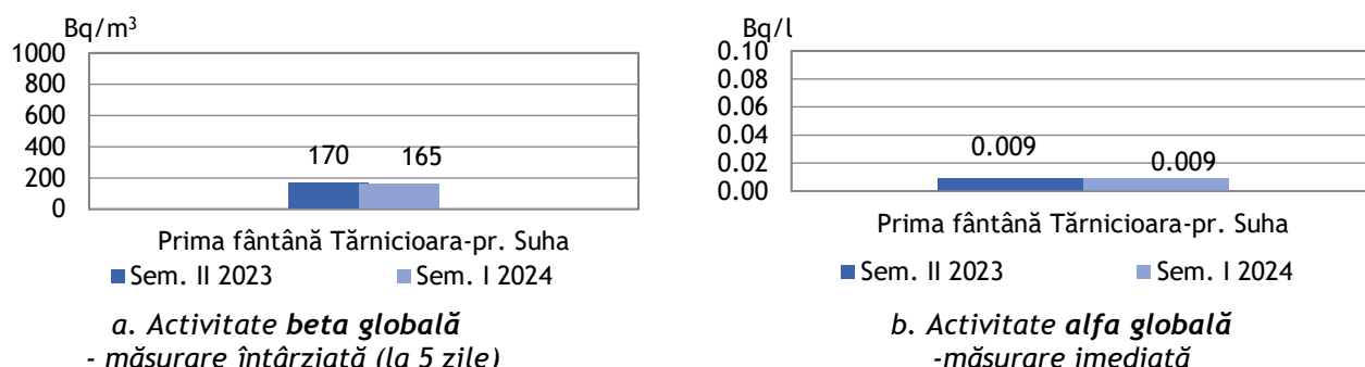
Fig. 2.4.2.2. Apă freatică - activități beta și alfa globale la probele prelevate în luna aprilie 2024 comparativ cu probele prelevate în perioade anterioare
