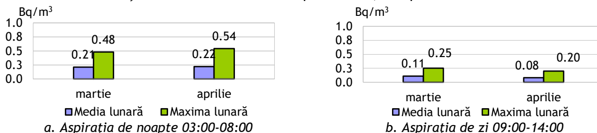
Fig. 2.2.2.2. Activități specifice ale Toronului (Rn-220) în atmosfera liberă - medii lunare și maxime zilnice în luna aprilie 2024, comparativ cu luna martie 2024
