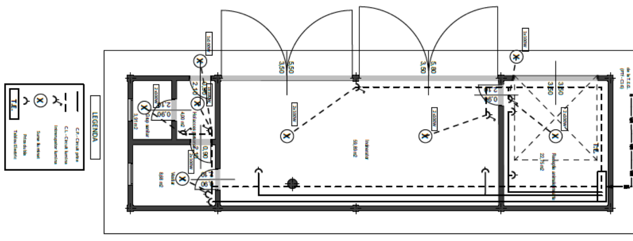
Plan detaliu clădire incinerator
